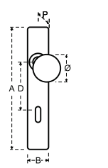
Pomolo decentrato girevole con placca Off-centre turnable knob with backplate
