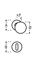
Pomolo fisso con rosetta e bocchetta Fixed knob with rose and lock profile
