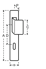
Maniglione reversibile con placca Reversible pull handle with backplate
