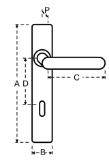
Maniglia con placca Handle with backplate
