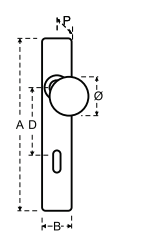
Pomolo decentrato girevole con placca Off-centre turnable knob with backplate
