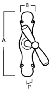
Cremonese a incasso Recessed cremone bolt Martellina con placca T handle with plate
