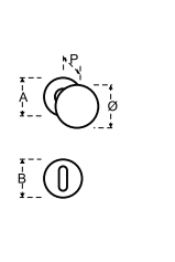
Pomolo decentrato girevole con rosetta e bocchetta Off-centre turnable knob with rose and lock profile
