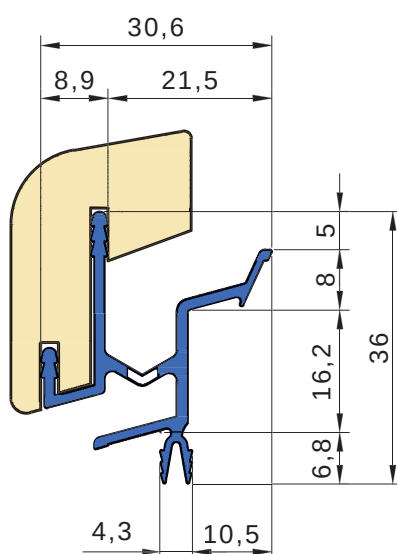
AL 2120 con terminali
