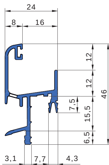
AL 2620 con terminali
