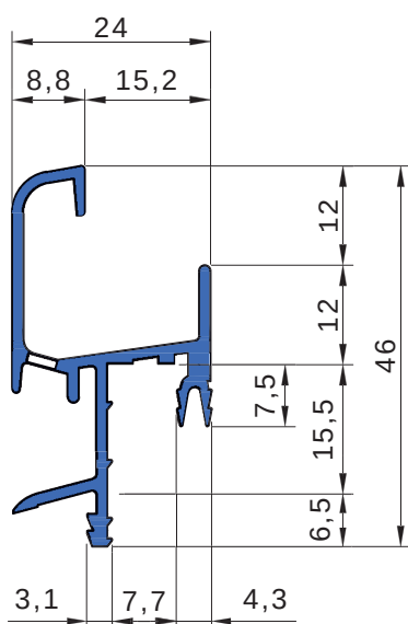
AL 1120 con terminali
