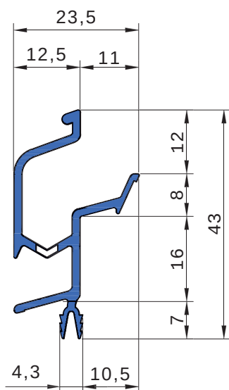
AL 2110 con terminali
