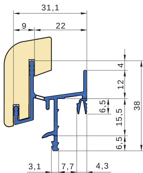
AL 1720 con terminali
