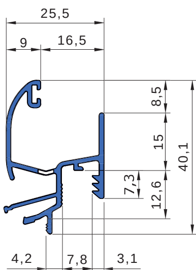
AL 3180 con terminali
