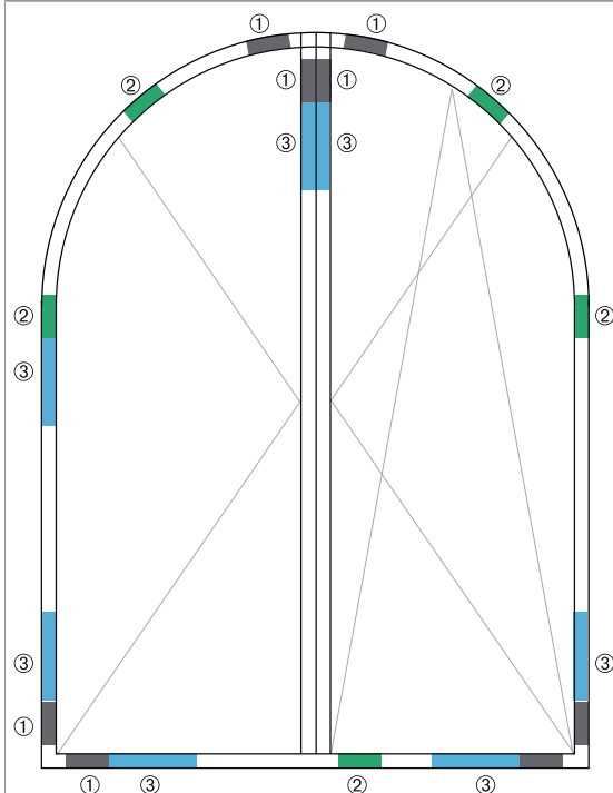
Serramento 2 ante ad arco, anta/ribalta
