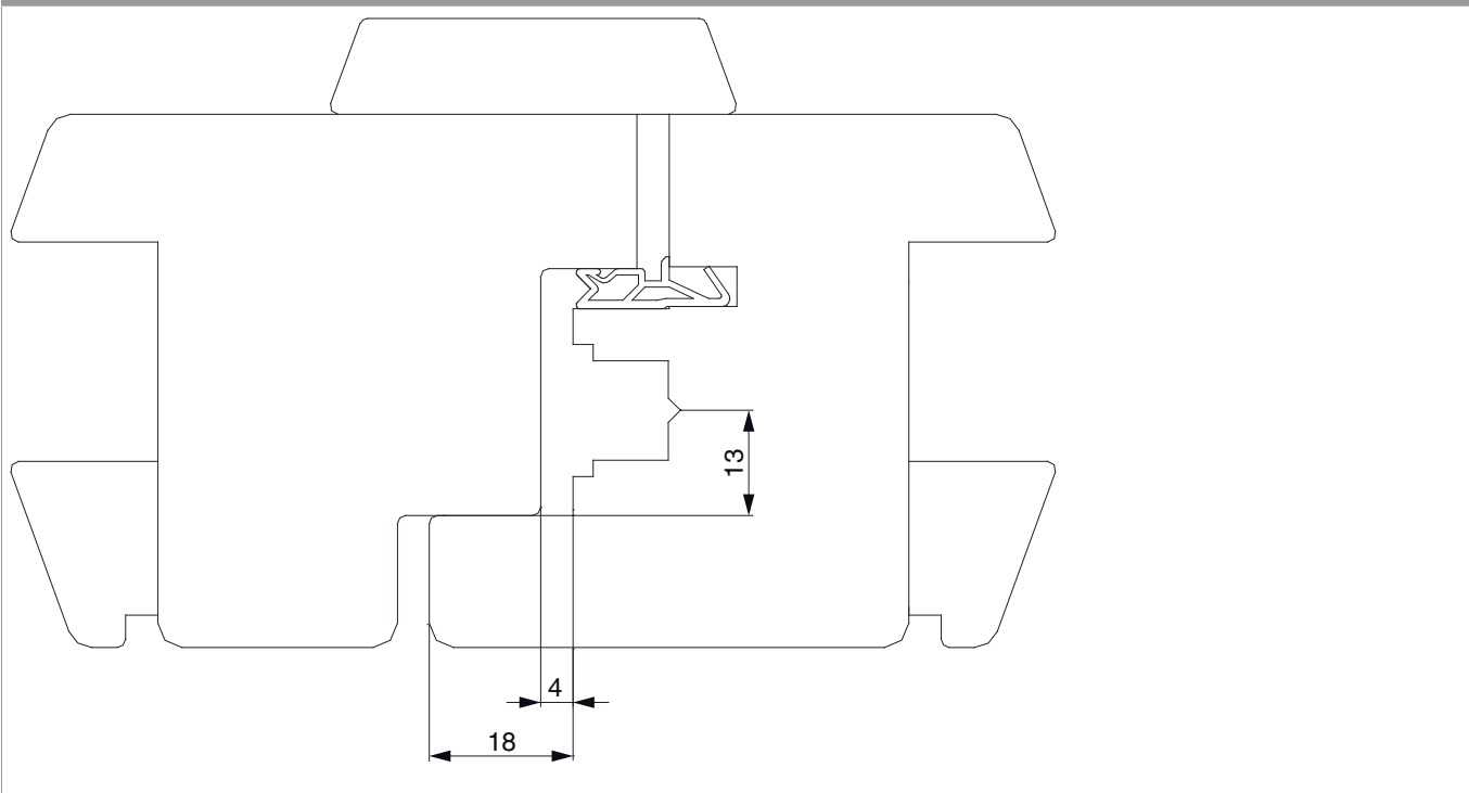
A4 scost.13 - 2 ante
