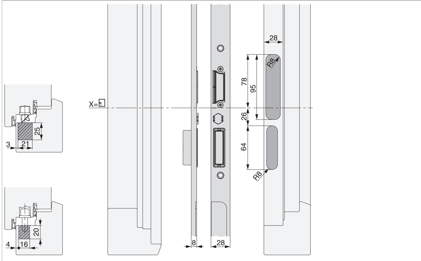
Dettaglio B
