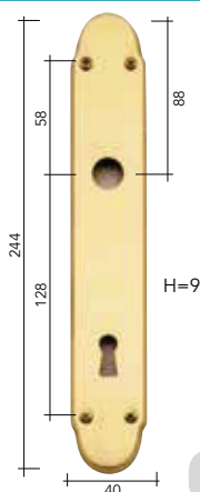
PLACCA PER MANIGLIA / PLATE FOR LEVER HANDLE
