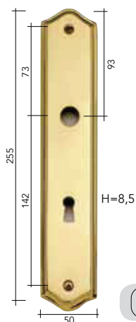
PLACCA PER MANIGLIA / PLATE FOR LEVER HANDLE
