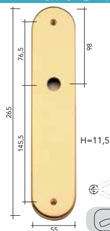
PLACCA PER MANIGLIA / PLATE FOR LEVER HANDLE
