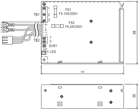
Alimentatore 230VAC - 13.8VDC - 3,6A
