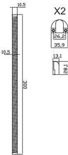
Passacavo flessibile da applicare L = mm 300 Apertura fino a 180°
